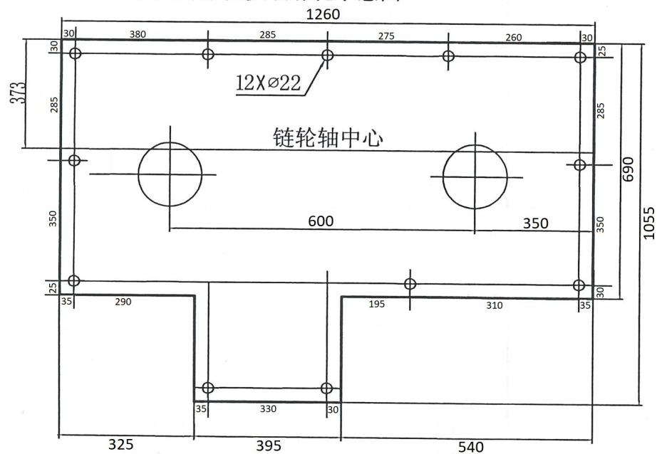
机座外形及安装螺孔示意图
